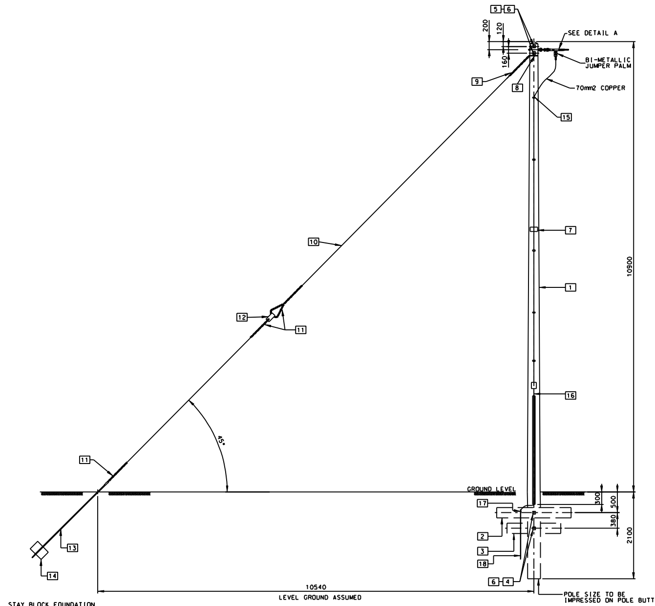
LONGITUDINAL ELEVATION
